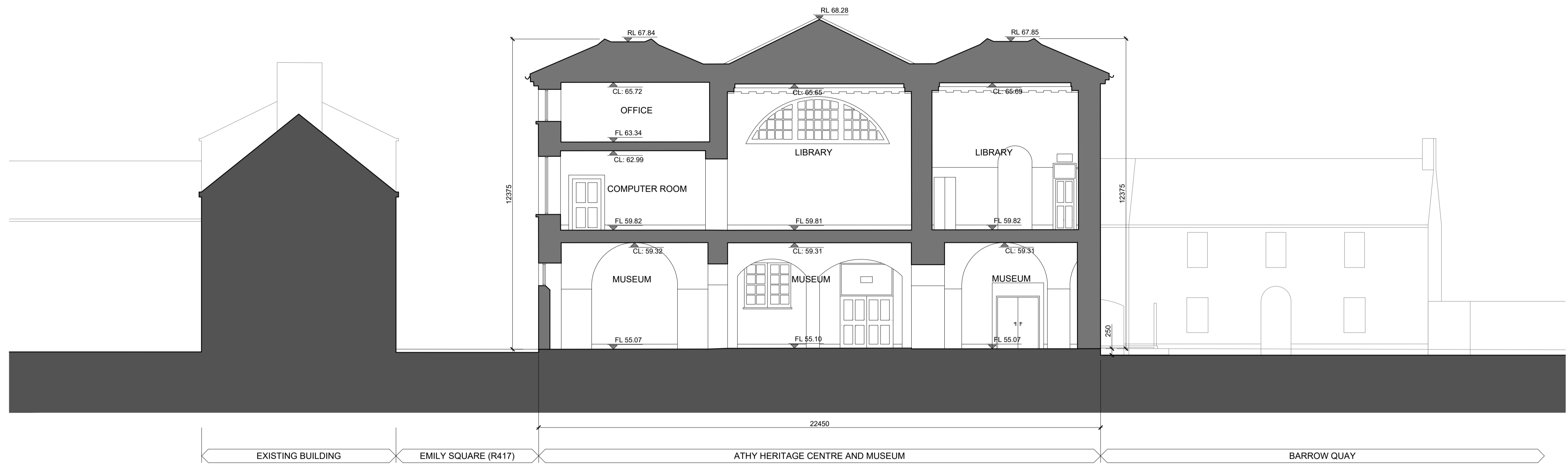
1 EXISTING SECTION A-A 1:100QA1, 1:200QA3
